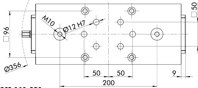
KSC3 160-280
