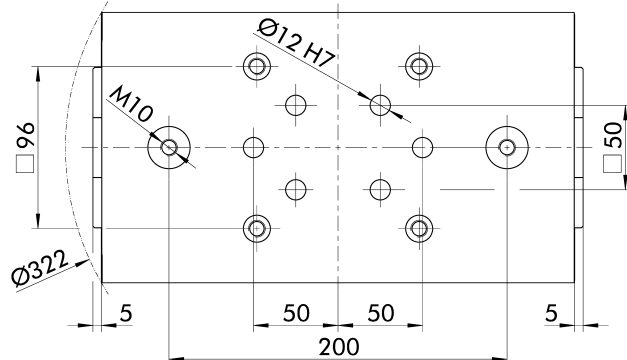
KSC3 160-280
