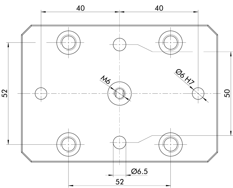
KSC mini 70-100
