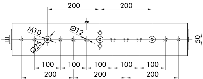
KSC-D 125-670
