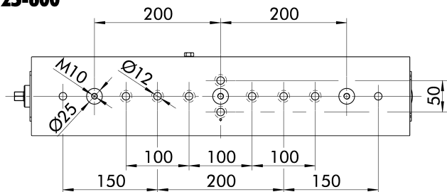
KSC-D 125-600
