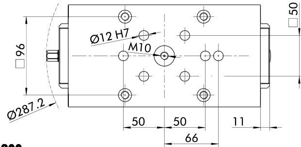
KSC3 125-235
