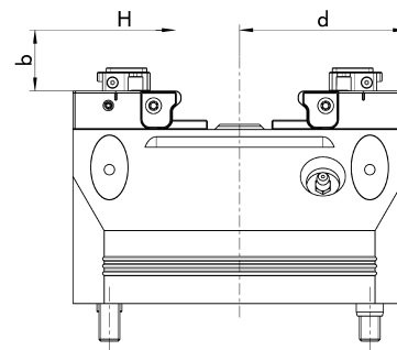
KSH3-BWA
